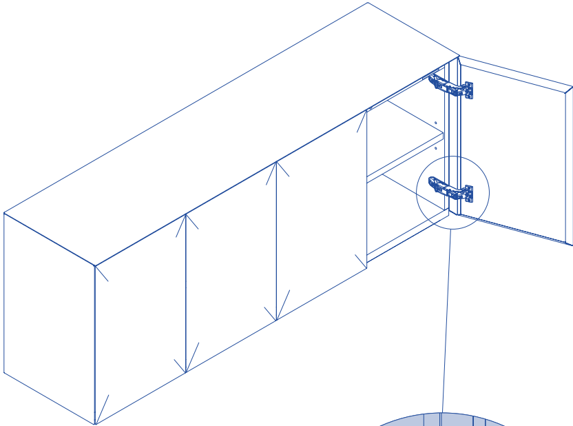
Blum CLIP top BLUMOTION 155°
